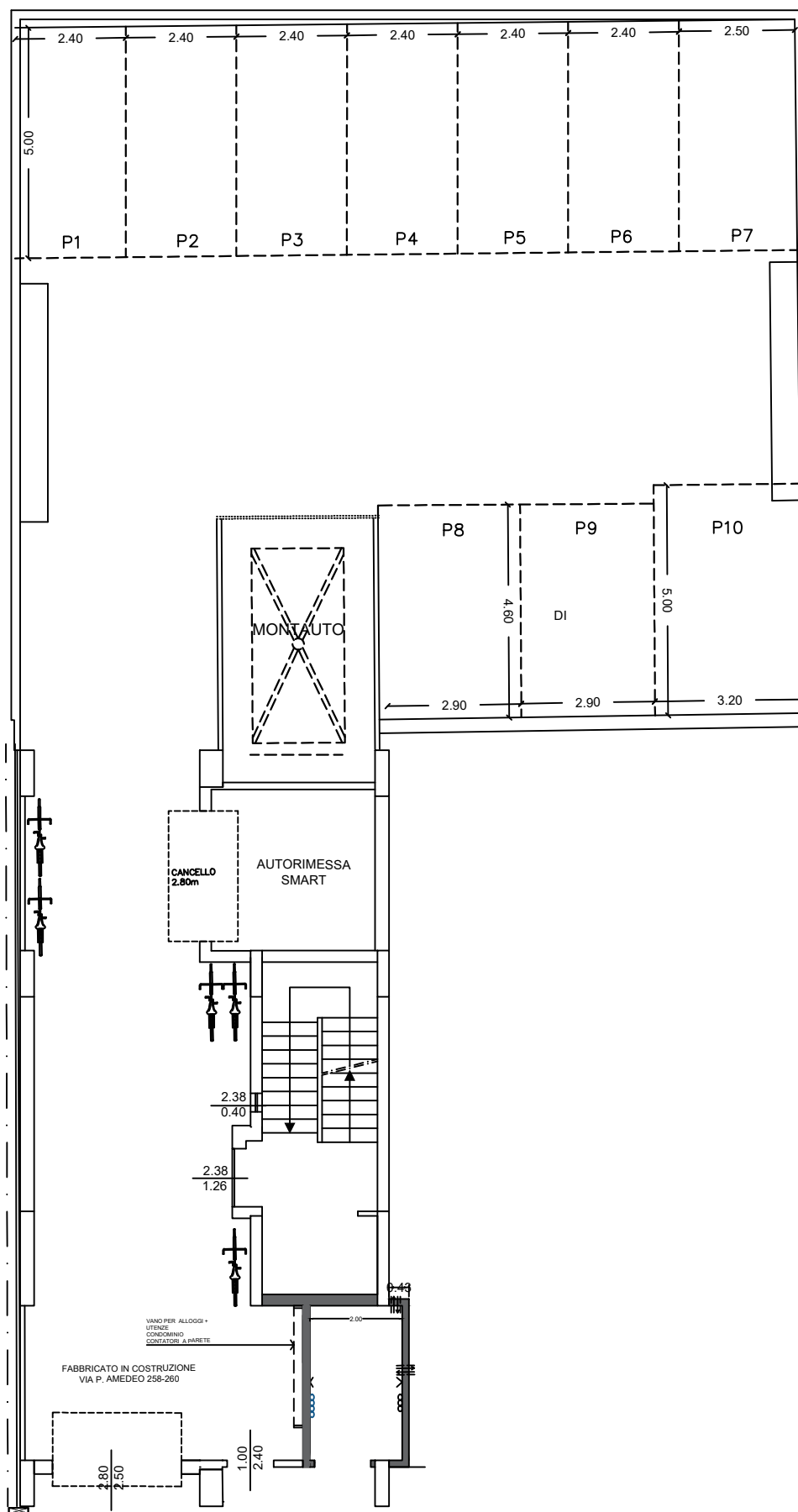
PLANIMETRIA PIANO TERRA Scala 1:100
